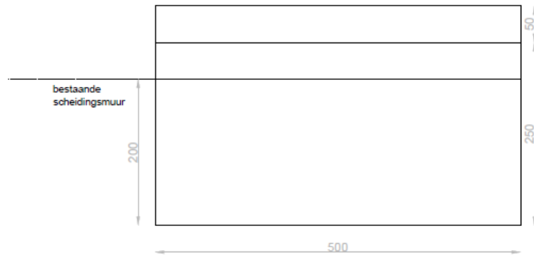
zijaanzicht rechts
