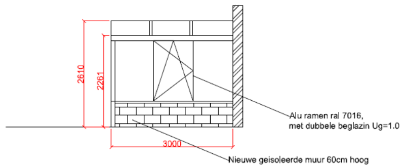
Vooraanzicht
