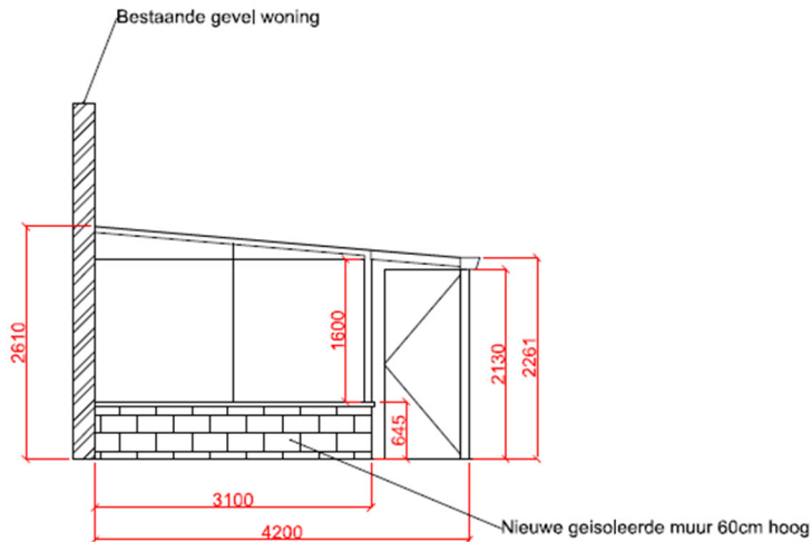
Zijaanzicht
