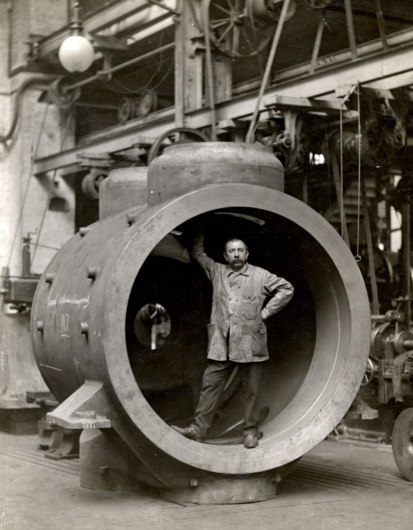
Cilinder van een stoommachine in machinewerkplaats van SEM-Carels in Gent. Foto door Joseph Buyens, ca. 1930. Collectie Industriemuseum
